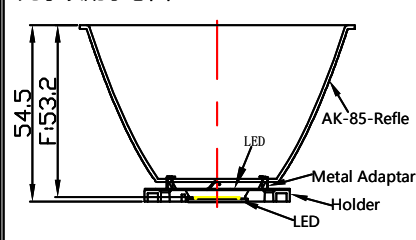
光学装配示意图
